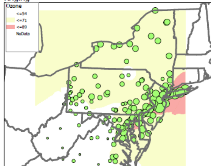
Kriging
